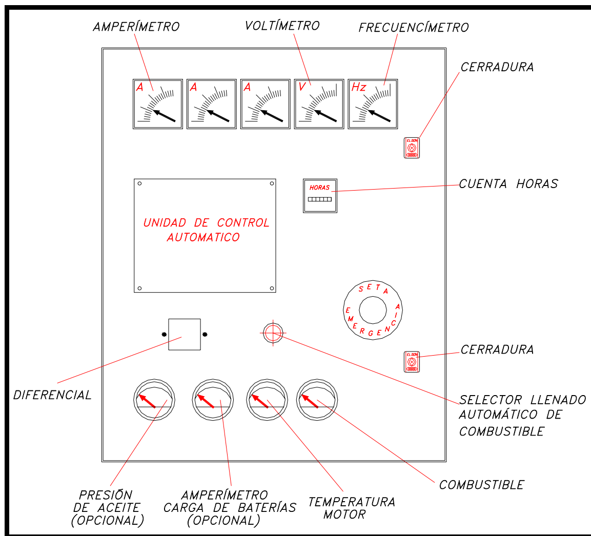
Imagen 6- Cuadro de Control genérico
