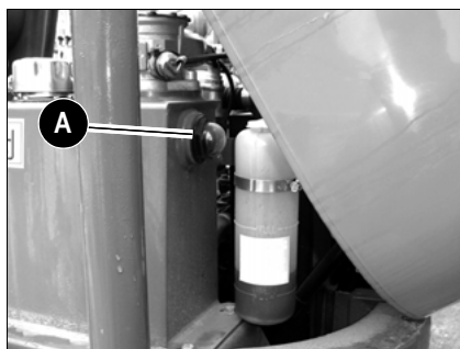
Fig. 42: Indicador del nivel de aceite en el depósito de
