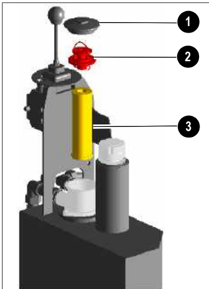
Fig. 46: Filtro de retorno-hidráulico
