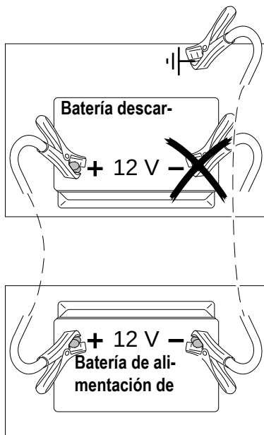
Fig. 28: Ayuda de arranque con cables de arranque
