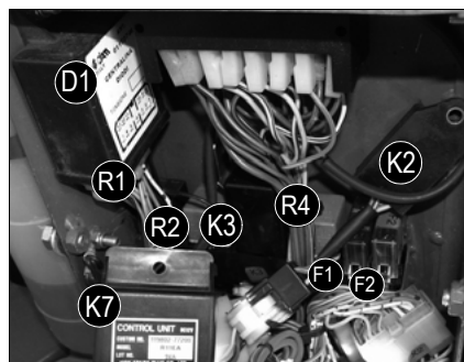
Fig. 57: Relés
