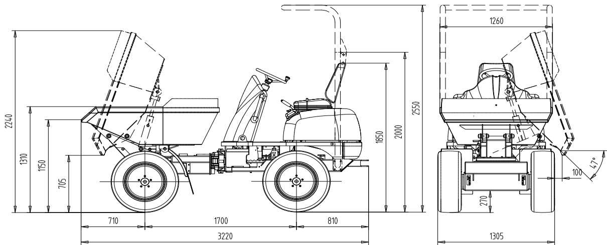
Fig. 55: Dimensiones del vehículo (modelo 1501S)
