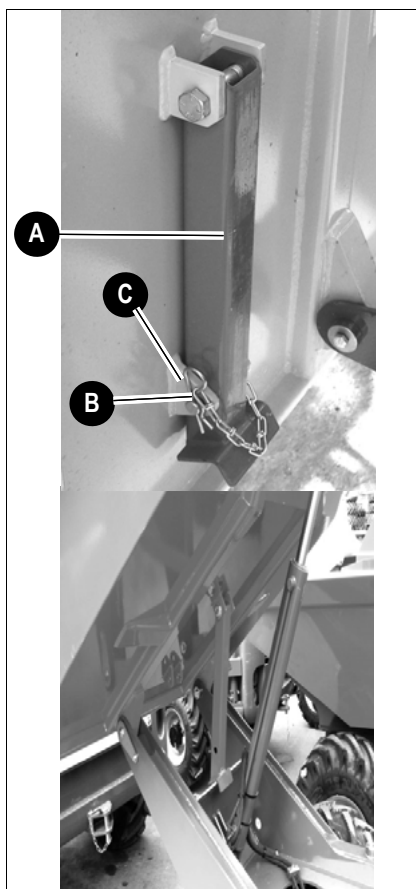
Fig. 29: Apoyos de mantenimiento
