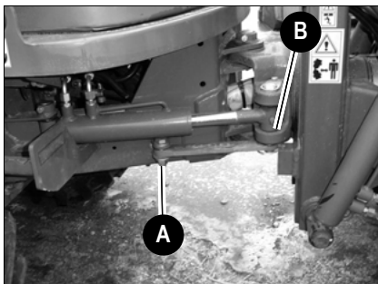
Fig. 50: Apoyos angulares
